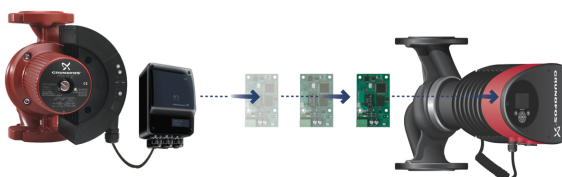
Fig. 66 Reuse of CIM module
